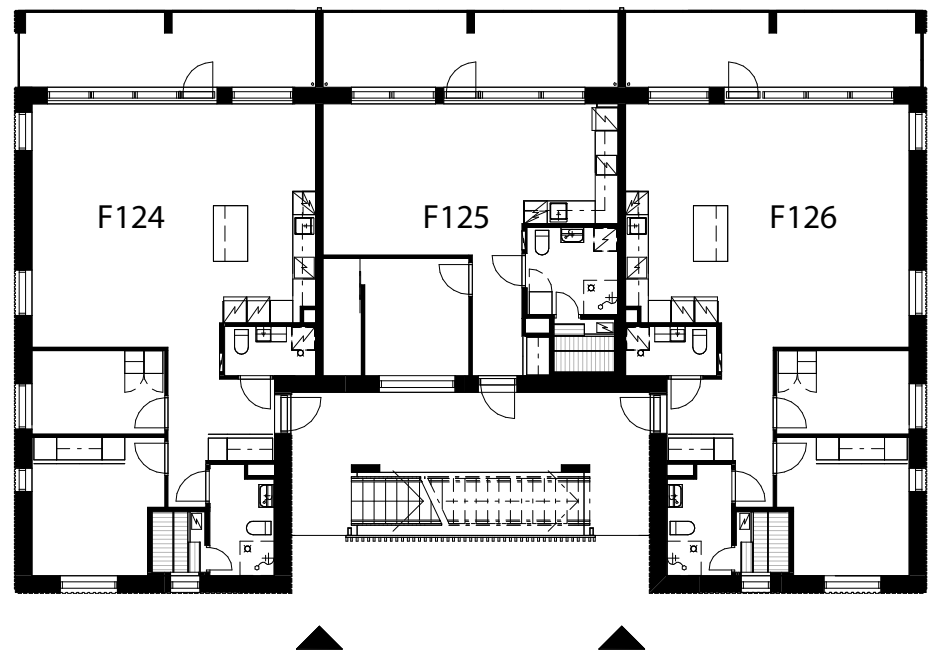
KERROS 2
