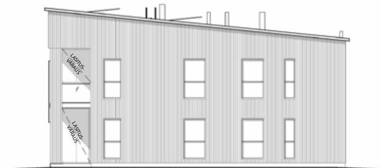
ETELÄÄN
